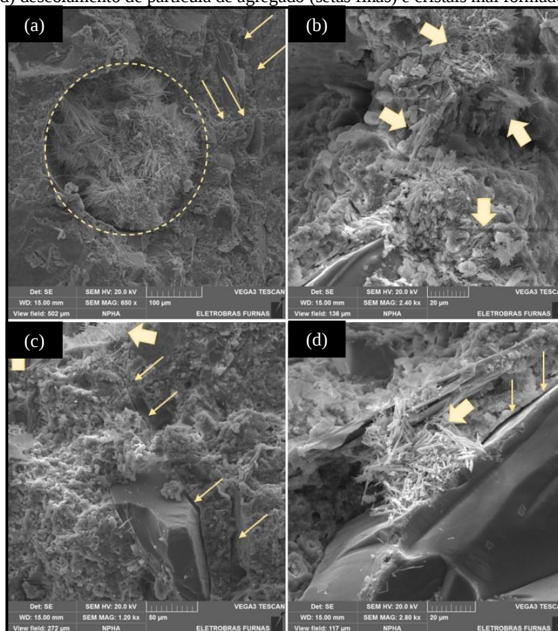
Figura 7 – Micrografias das argamassas aos 365 dias: a) cristais aciculares formados dentro de um poro; b) formações massivas na matriz cimentícia (setas largas); c) descolamento de partícula de agregado e fissura desencadeada ao longo da pasta de cimento (setas finas), além de cristais de etringita no entorno e em poro próximo (setas largas); d) descolamento de partícula de agregado (setas finas) e cristais mal formados (setas largas).
