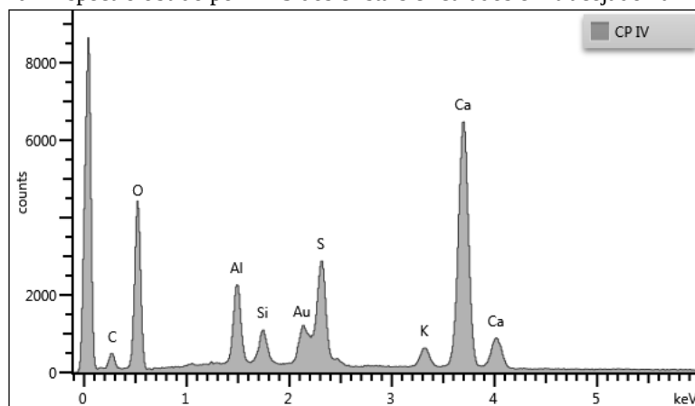
Figura 10 – Espectro obtido por EDS dos cristais circulados em tracejado na Figura 9d.
