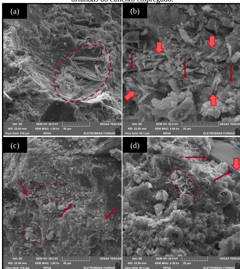
Figura 9 – Micrografias dos concretos aos 365 dias: a) deposição de cristais mal formados em poro; b) fissura na pasta (setas finas) acompanhada e formações de etringita no entorno (setas maiores); c) fissura observada no concreto (setas finas), no entorno com o agregado, e presença constante de cristais de etringita na matriz cimentícia (círculos tracejados); d) etringita formada nas proximidades do agregado, além de partículas de cinza volante oriundas do cimento empregado.
