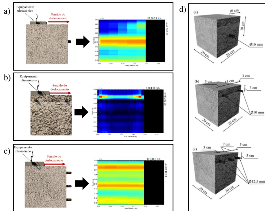
Figura 5 - Detecção de barras de aço no interior dos CPs através de tomografia utilizando VPU de a) uma barra; b) duas barras; c) três barras; d) detalhes dos CPs ensaiados
