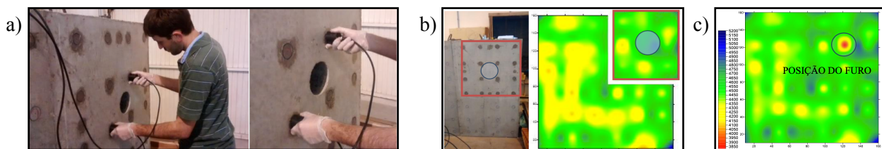
Figura 2 - Ensaio não destrutivo de interpolação de velocidades de pulsos ultrassônicos em parede de 1,70 m x 170 m x 0,6 m a) leitura indireta; b) resultado gráfico das leituras antes do furo, ensaio 2; c) resultado gráfico das leitura depois do furo, ensaio 2
