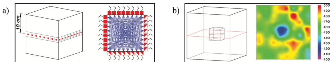
Figura 3 - a) Leituras de ultrassom realizadas em uma determinada altura de um corpo de prova (CP) de concreto contendo um objeto de menor densidade no interior; b) tomografia ultrassônica do CP
