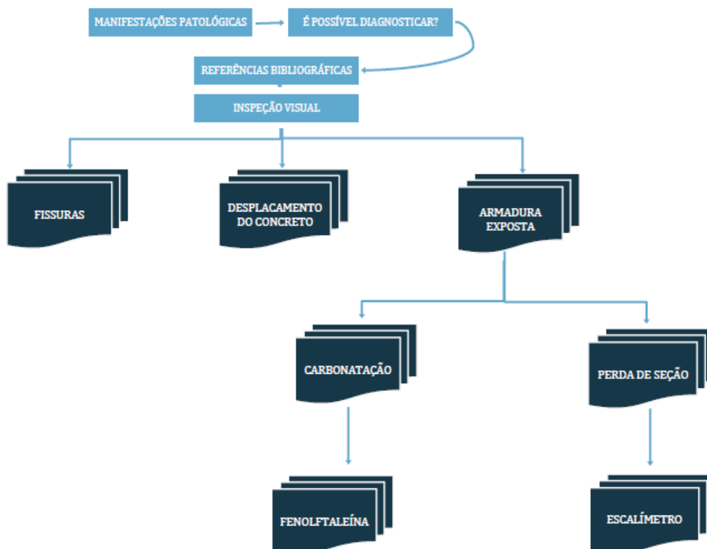
Figura 2 – Fluxograma da análise de corrosão em estruturas
