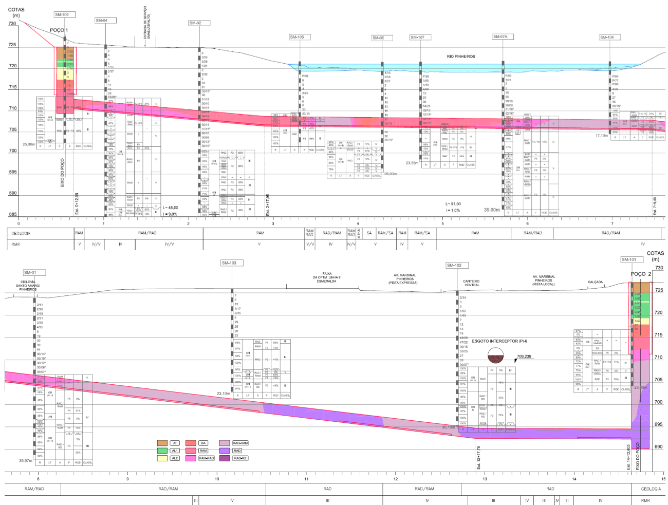
Figura 2 - Mapeamento Geológico dos Poços e Túnel.
