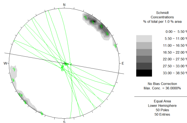
Figura 5 - Projeção estereográfica com dados das fraturas obtidas nos mapeamentos de frente.
