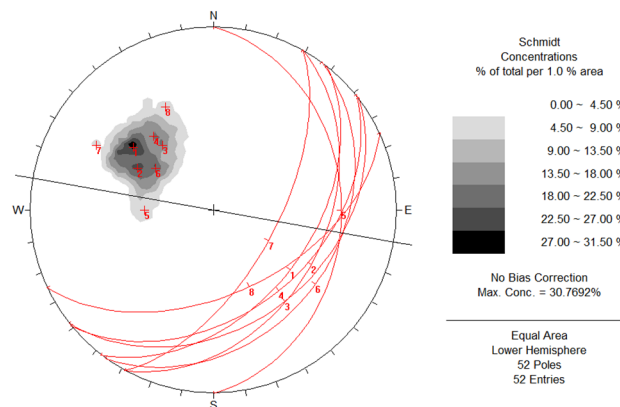
Figura 4 - Estereograma com dados da foliação obtidos nos mapeamentos.
