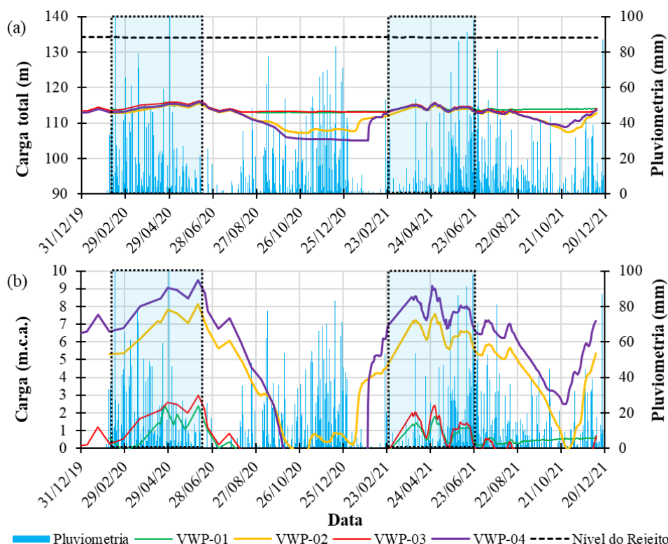
Figura 2. Variação ao longo do tempo de (a) Cargas totais e (b) Poropressões monitoradas.
