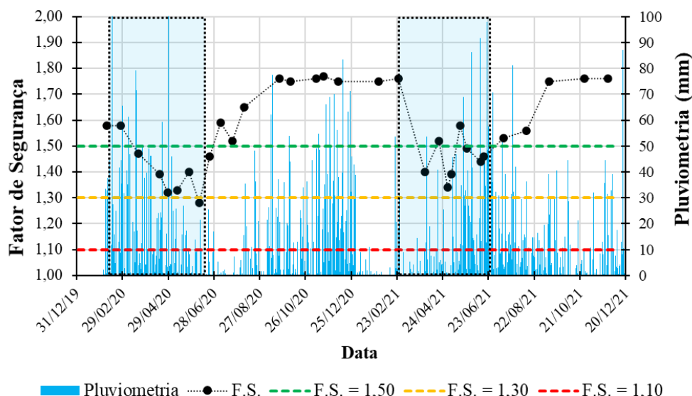
Figura 4. Resumo das análises de estabilidade elaboradas.
