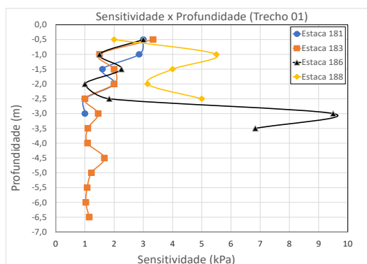
Figura 16. Sensitividade x profundidade trecho 01.
