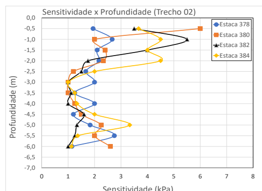
Figura 17. Sensitividade x prof. trecho 02.
