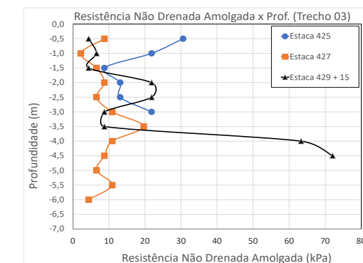
Figura 15. Resistência não drenada amolgada x profundidade para trecho 03.
