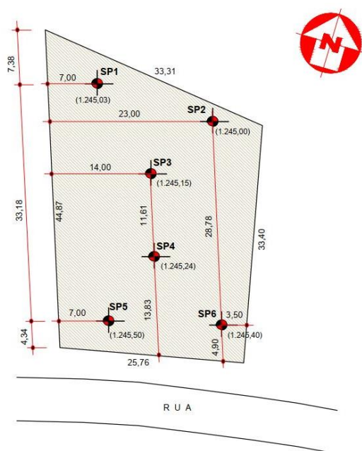
Figura 10. Localização dos furos da 1ª campanha de sondagem.
