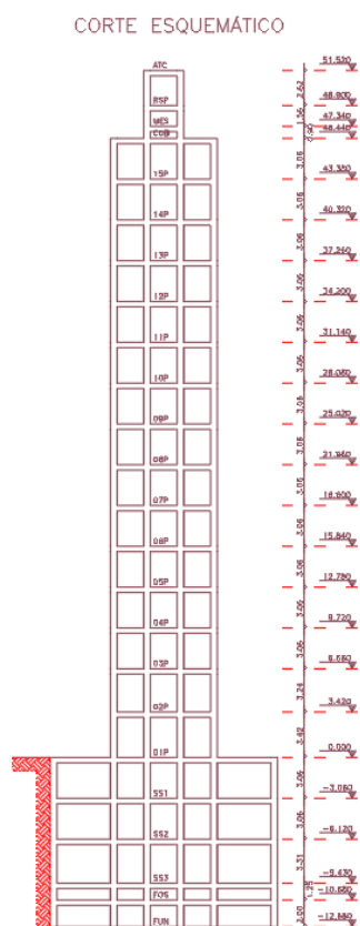
Figura 8. Vista em corte do empreendimento. (FHE, 2019).
