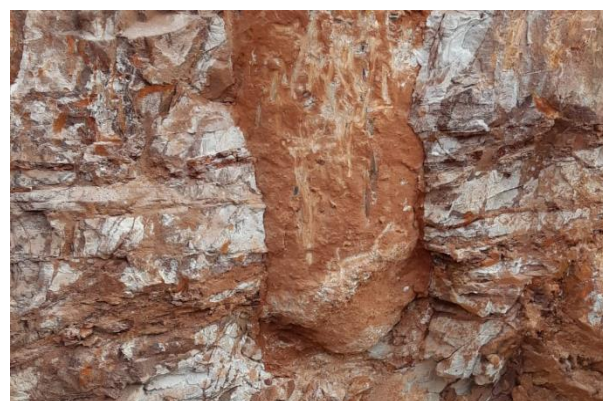
Figura 15. Ponta da estaca hélice contínua paralisada antes da cota prevista em função da resistência do material.
