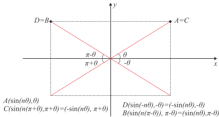
Figura 2: simetrias do ponto A(\sin(n\theta), \theta) com n ímpar.
