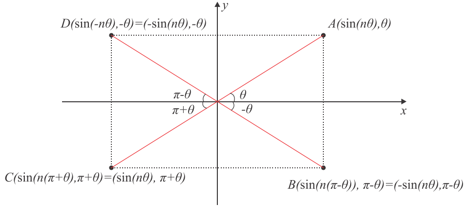
Figura 1: simetrias do ponto A(\sin(n\theta), \theta) com n par.
