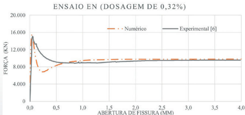
► Figura 6 Força por abertura de fissura com reforço de 0,32% de fibra no ensaio EN 14651
