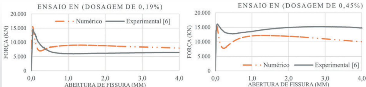
► Figura 7 Força por abertura de fissura com reforço de 0,19% e 0,45% de fibra no ensaio EN 14561
